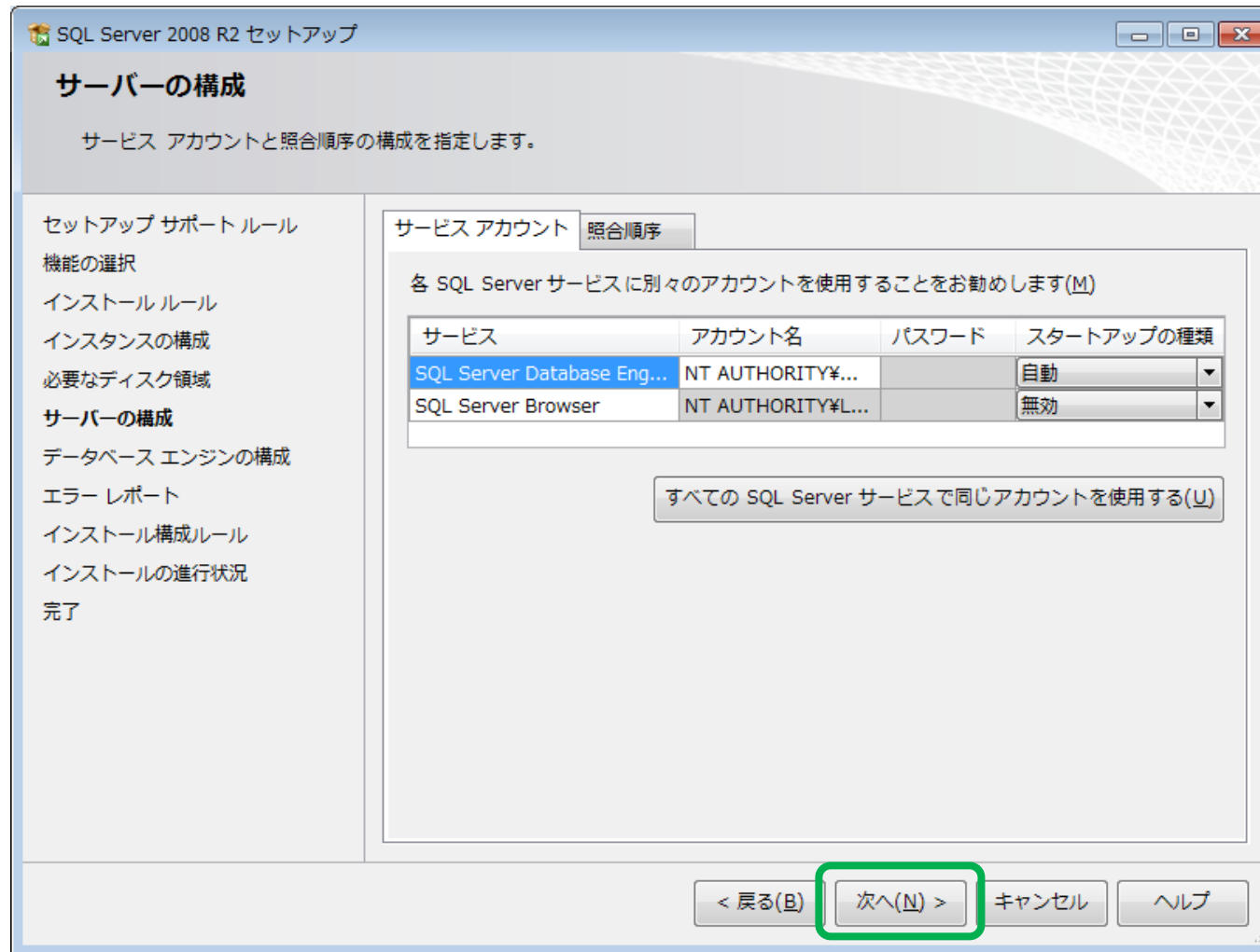
図 20 サーバーの構成
