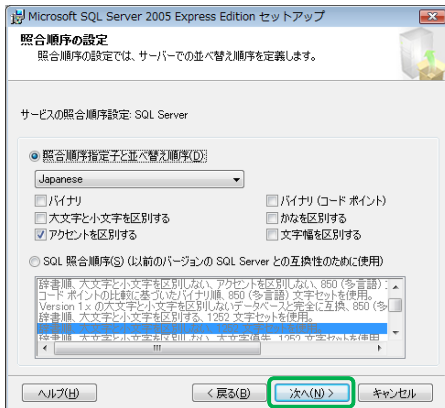
図 14 照合順序の設定
