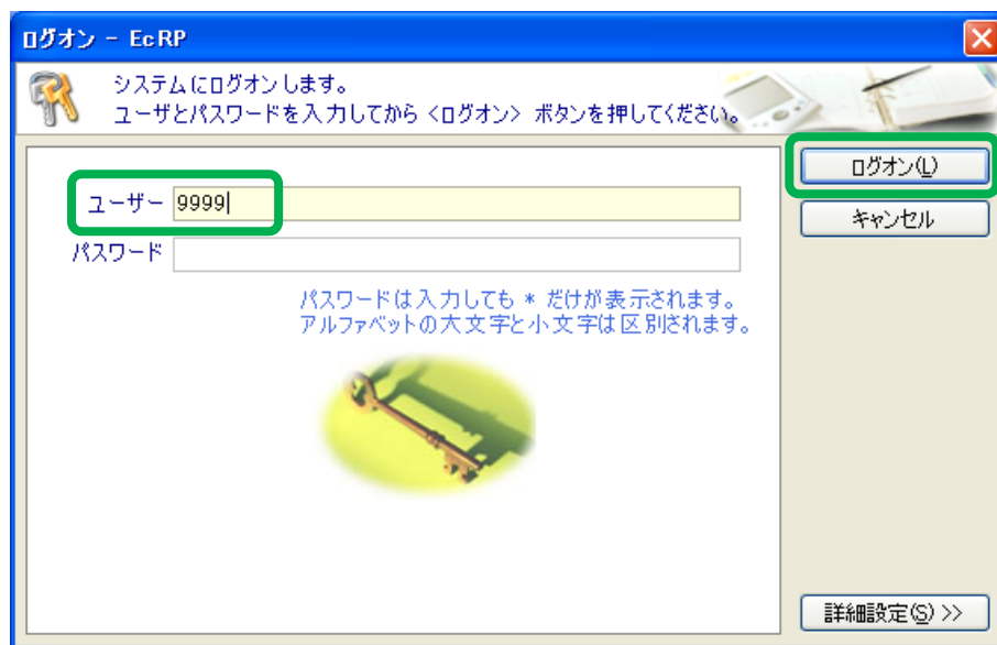
図 31 ログオン
