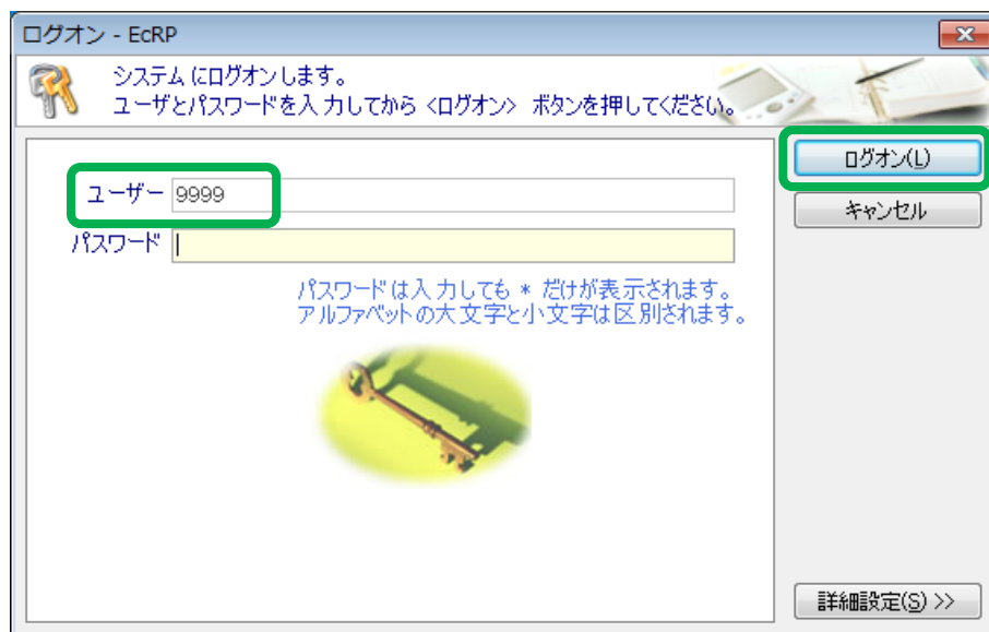
図 23 ログオン
